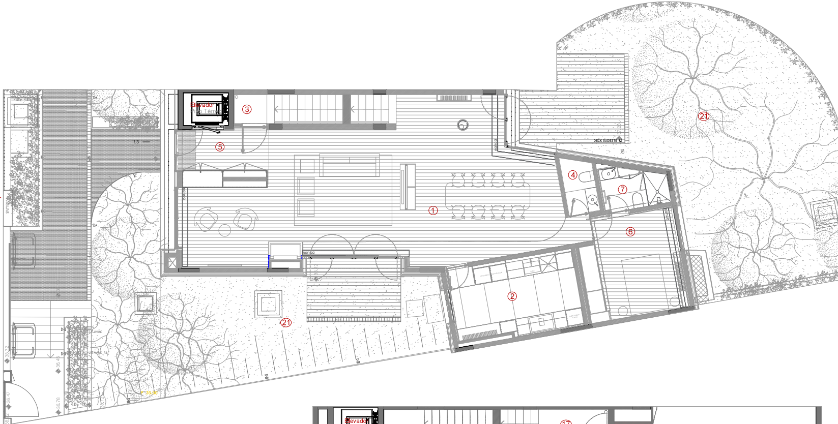
PISO TÉRREO
